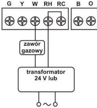
dla 2 przewodowego 24V systemu ogrzewania
