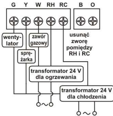
dla 5 przewodowego (z 2 trafo) systemu ogrzewania i chłodzenia
