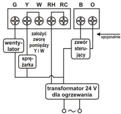
dla 1 stopniowego systemu pompy ciepła
