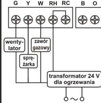
dla 4 przewodowego systemu chłodzenia i ogrzewania
