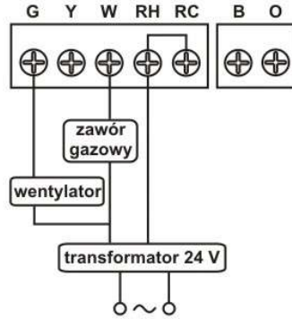
dla 3 przewodowego systemu ogrzewania, jeżeli 3 przew. steruje wentylatorem
